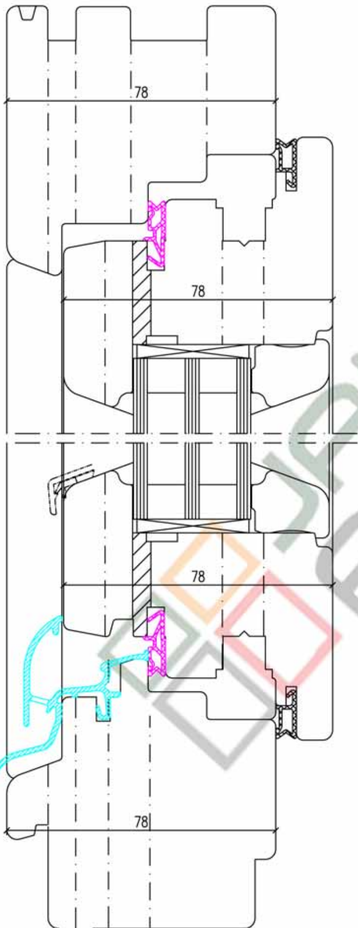
Metszet: A - A
